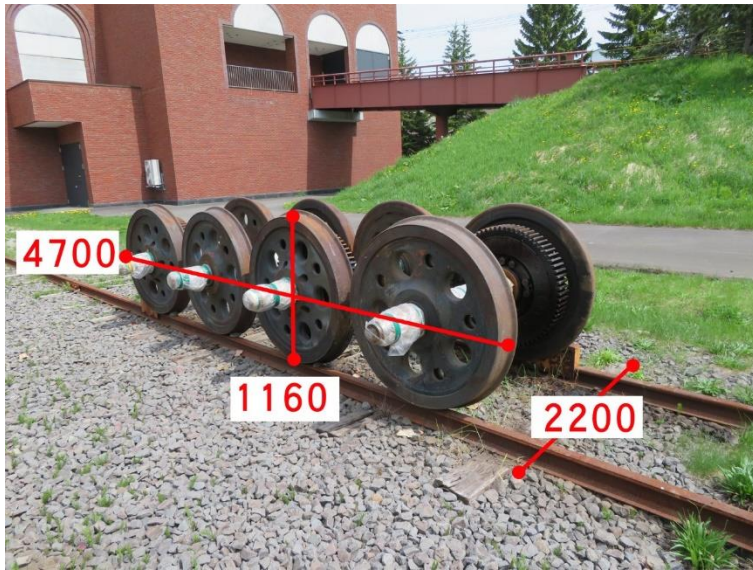
④動輪 4 対
