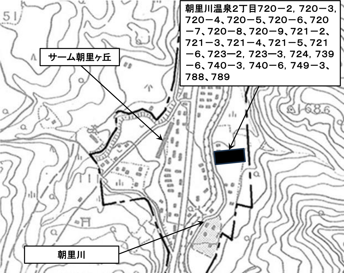
位置図
