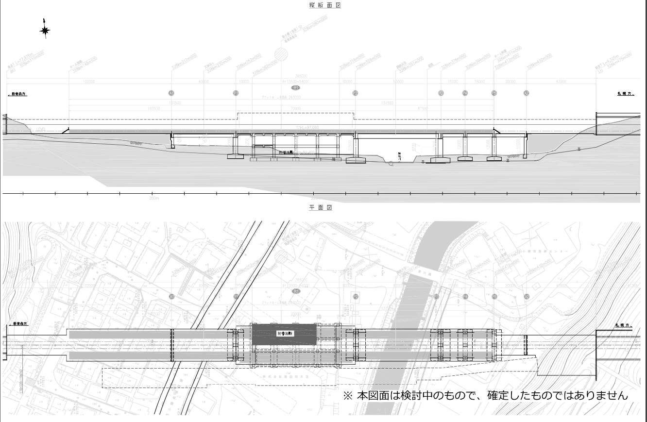
新小樽（仮称）駅 施設配置図（案）
