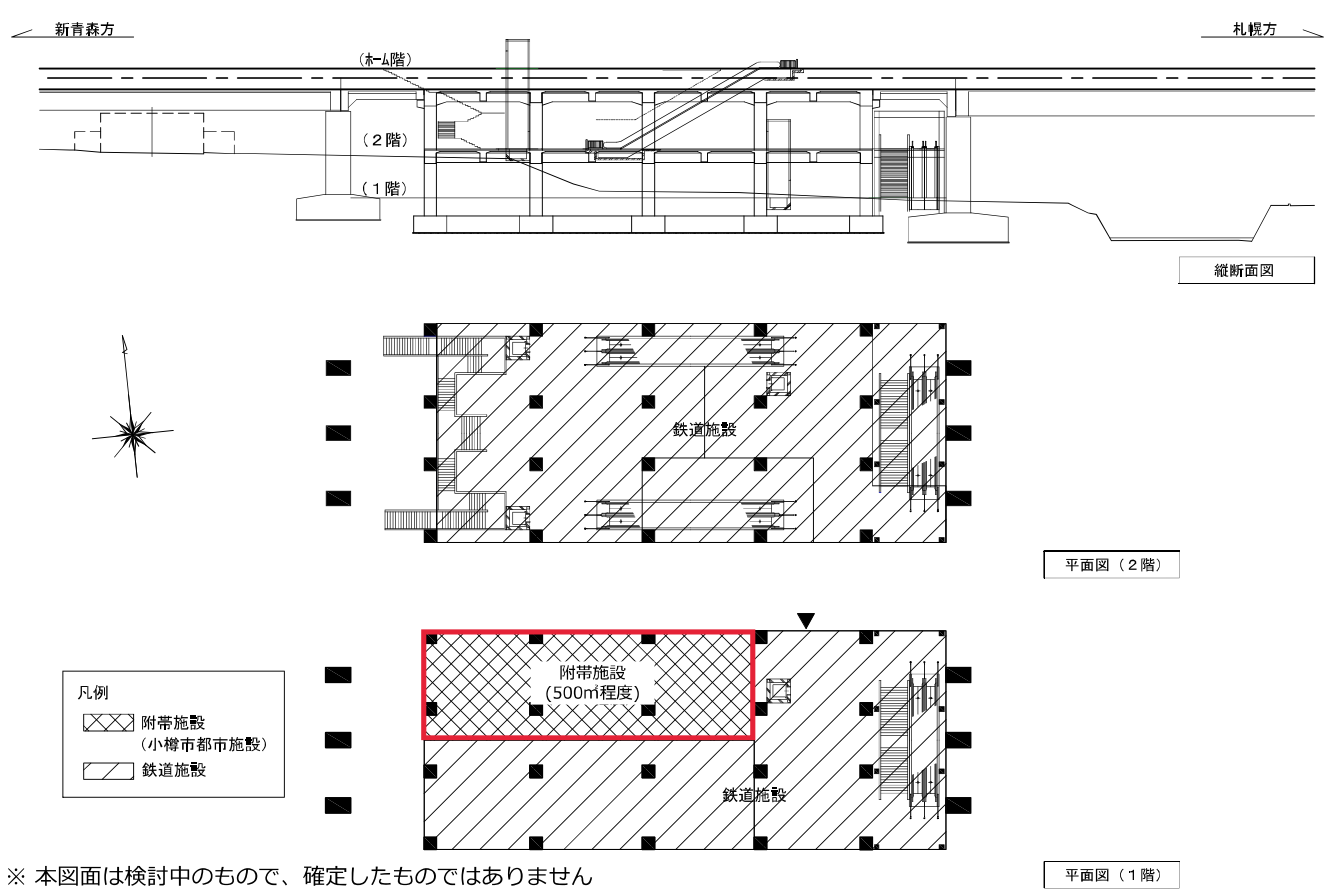
新小樽（仮称）駅施設配置図（案）
