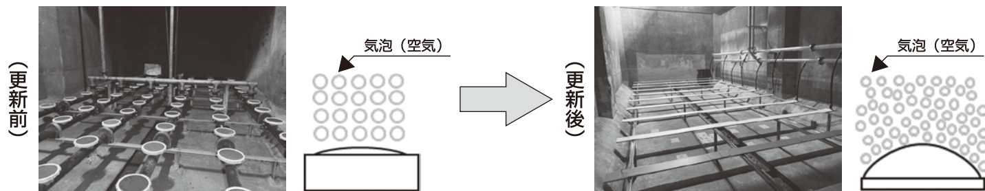
【写真・断面図】散気装置
