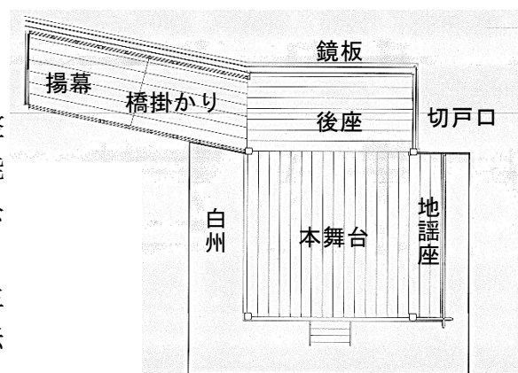
旧岡崎家能舞台平面図
