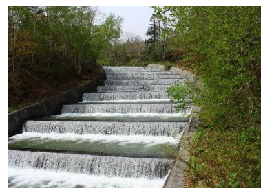
奥沢水源地 階段式溢流路
