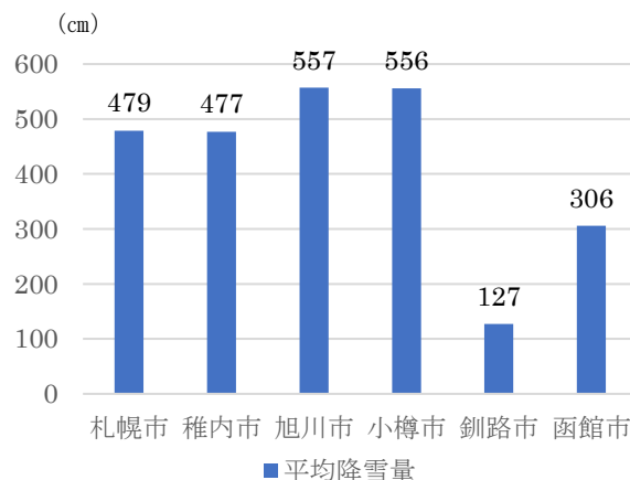
道内主要都市の降雪量
